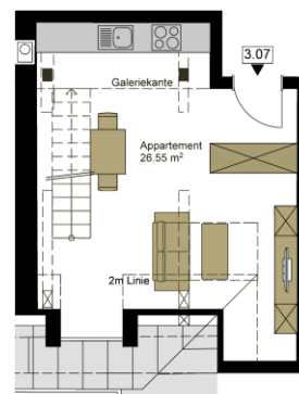
Grundriss 1. Dachgeschoss
