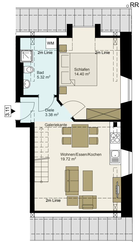
Grundriss 1. Dachgeschoss
