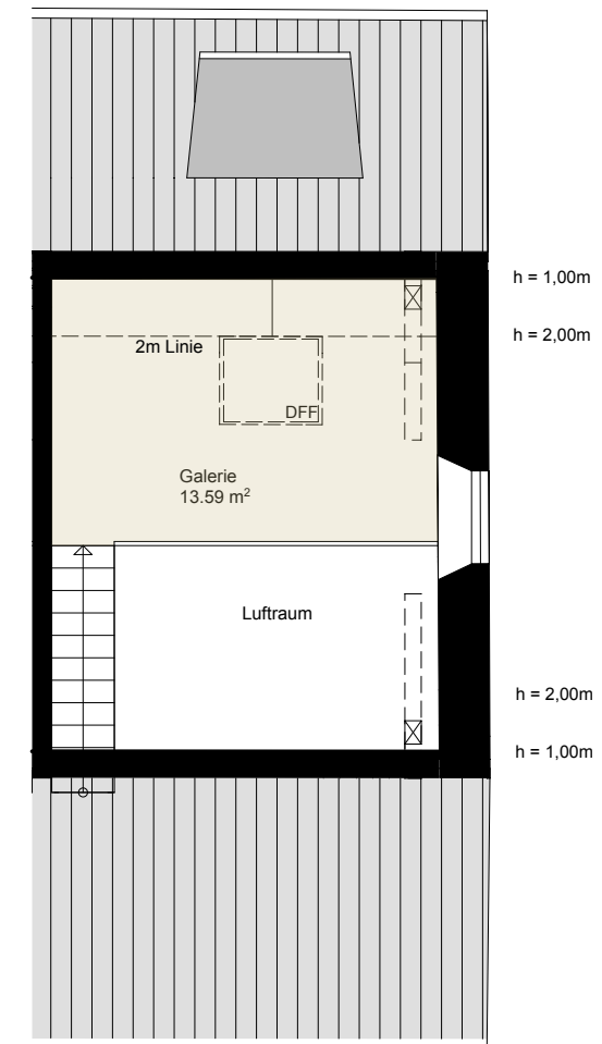
Grundriss 2. Dachgeschoss
