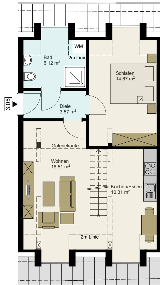
Grundriss 1. Dachgeschoss
